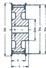
Ausf. Type 6WF
