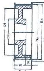
Ausf. Type 5WF
