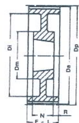
Ausf. Type 9W
