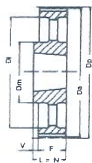
Ausf. Type 8A
