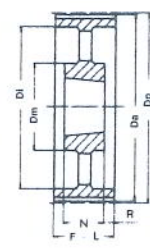
Ausf. Type 9A
