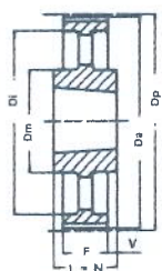
Ausf. Type 7A
