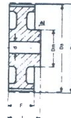
Ausf. Type 6W
