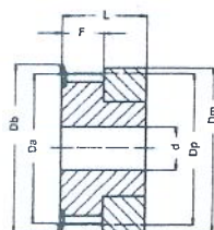
Ausf. Type 1F
