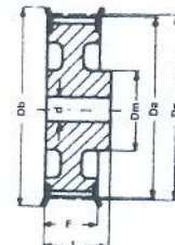
Ausf. Type 6WF
