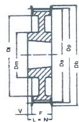
Ausf. Type 8WF
