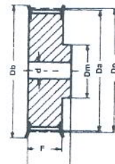
Ausf. Type 6F
