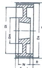
Ausf. Type 9W
