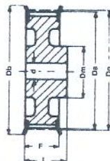
Ausf. Type 6WF
