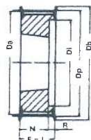
Ausf. Type 5F
