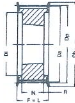
Ausf. Type 4F
